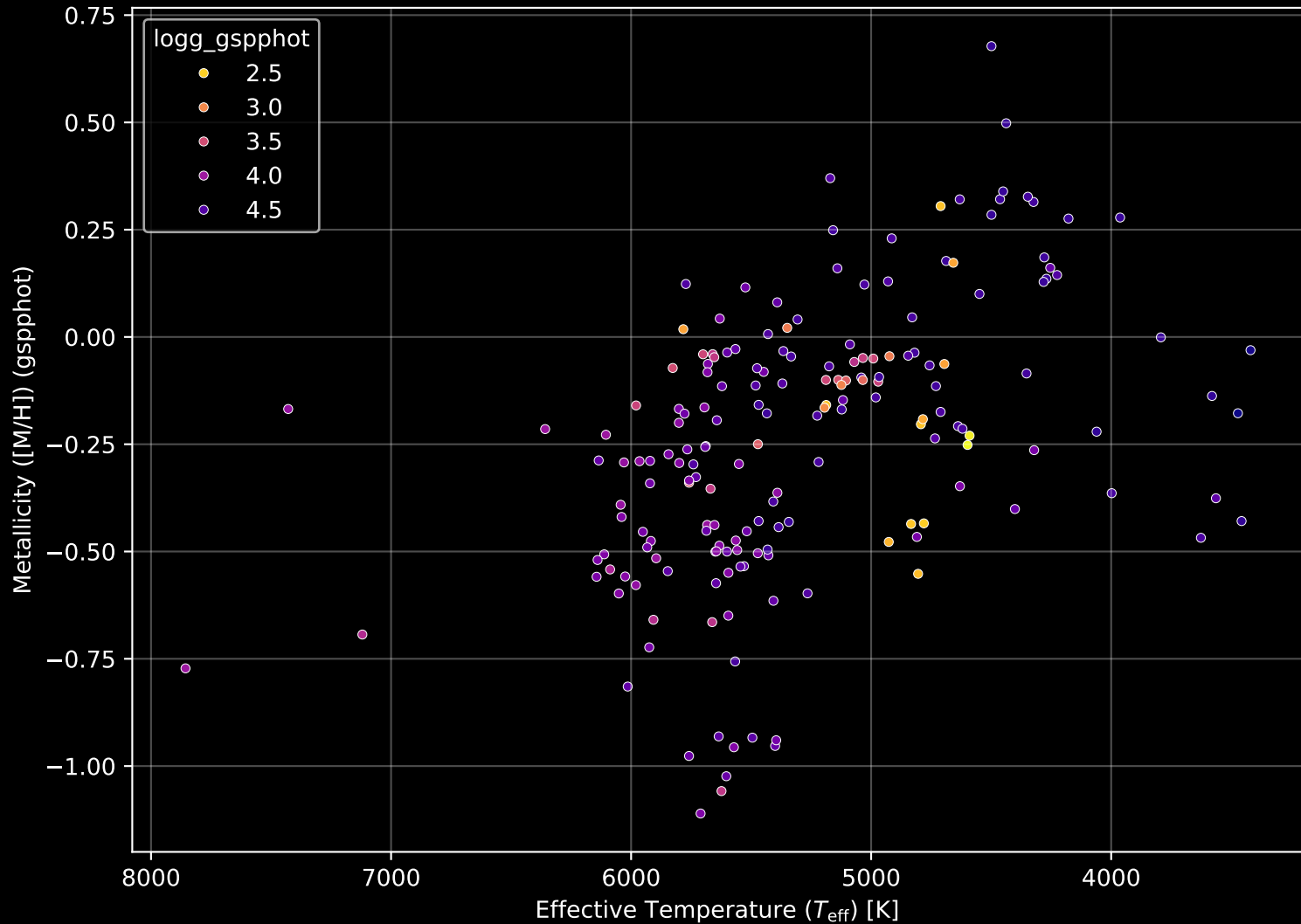
APOGEE DR17 Field: [224+49_btx] Stellar Population Parameters (n= 185)
